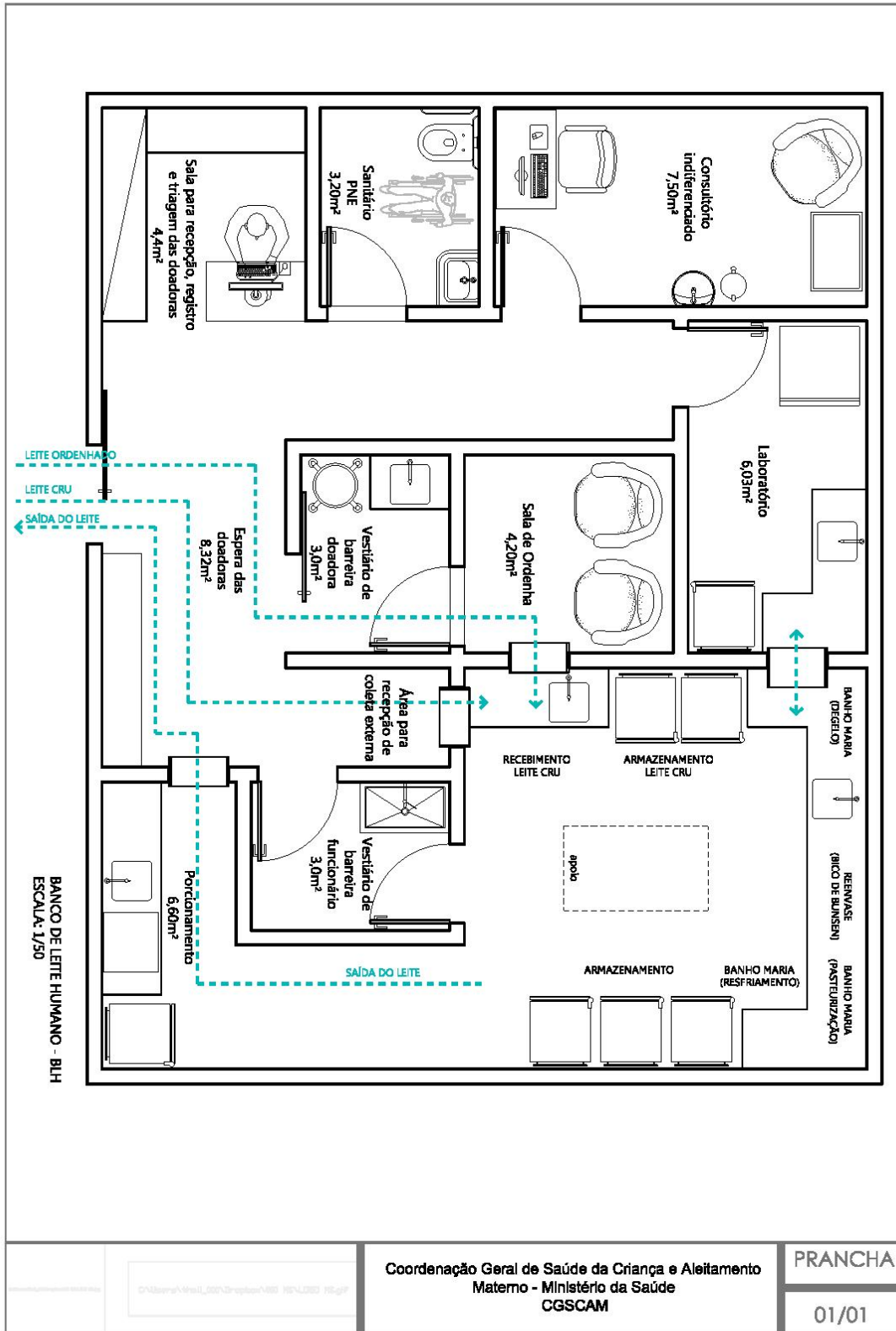
Planta del BLH del Complejo Hospitalario Dr. Arnulfo Arias Madrid, Ciudad de Panamá
