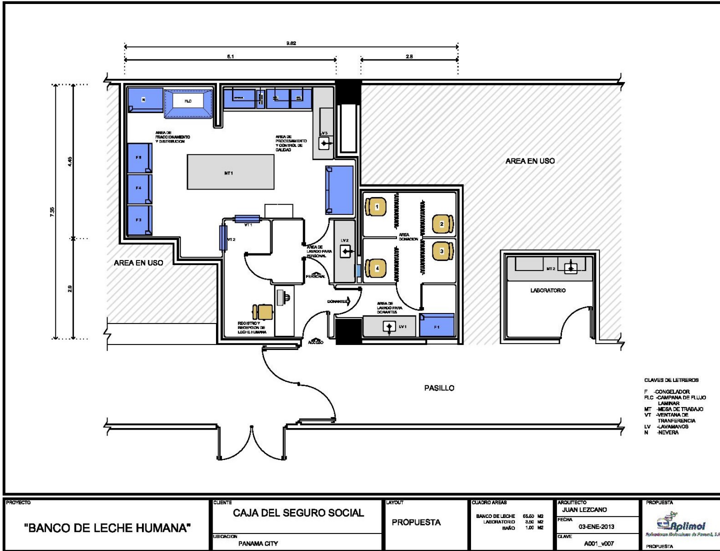
Planta del BLH del Hospital de Fusagasugá, Colombia
